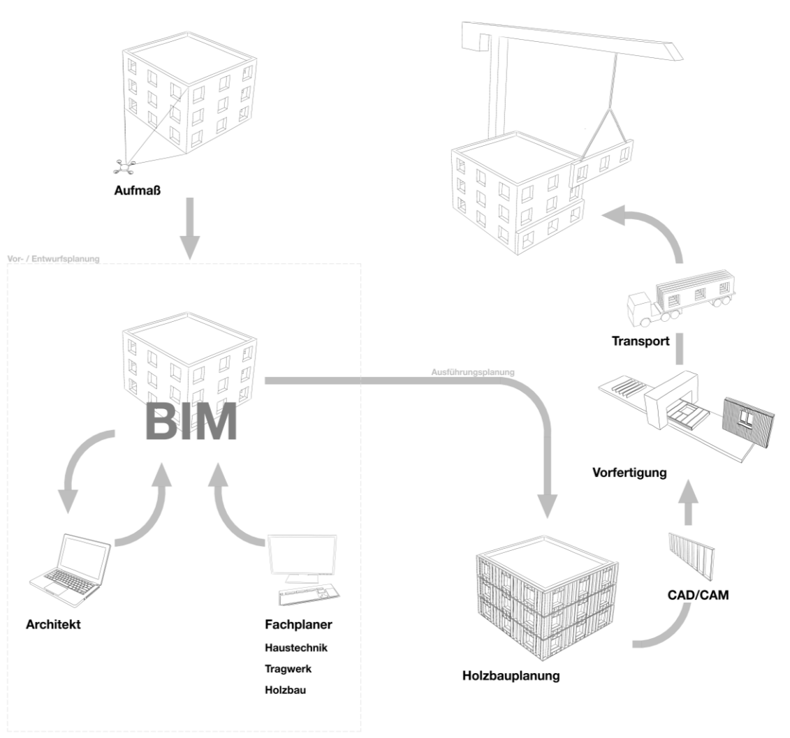
Abbildung 2: TES Prozessgrafik: Aus dem digitalen Aufmaß entsteht das Bestandsmodell, welches die Grundlage für den folgenden, integralen Planungsprozess bildet. Vom Aufmaß bis zur Montage folgt die Modernisierung mit dem Timber Element System (TES) einem systematischen, digitalen Workflow.
