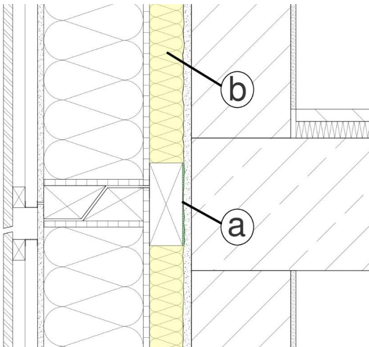
Abbildung 7: Ausgleich der vorhandenen Toleranzen am Bestandsgebäude (a) Die Montagebalken werden durch Abstandhalter ausgerichtet (b) Der verbleibende Hohlraum wird vor Anbringen der Elemente mit Mineralwolle gefüllt
